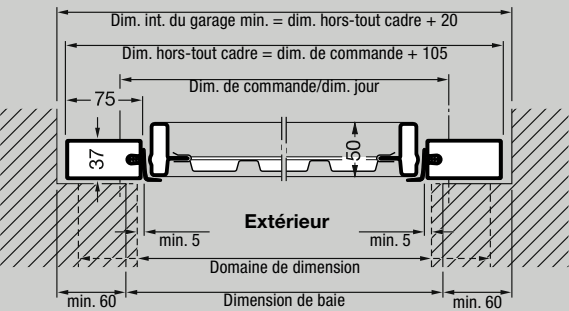
Coupe horizontale
