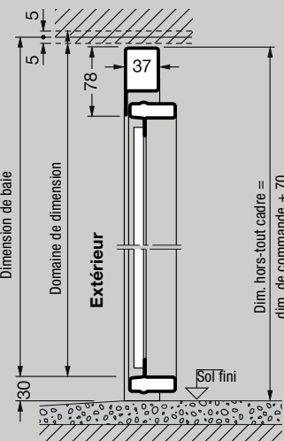
Coupe verticale
