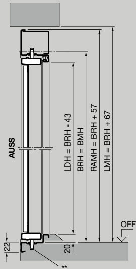
Coupe verticale – Porte avec seuil
