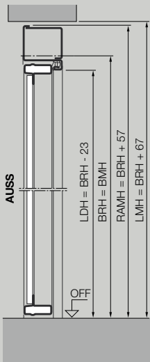
Coupe verticale – Porte sans seuil
