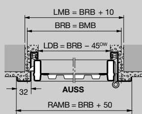
Coupe horizontale
