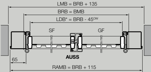
Coupe horizontale
