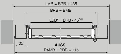
Coupe horizontale
